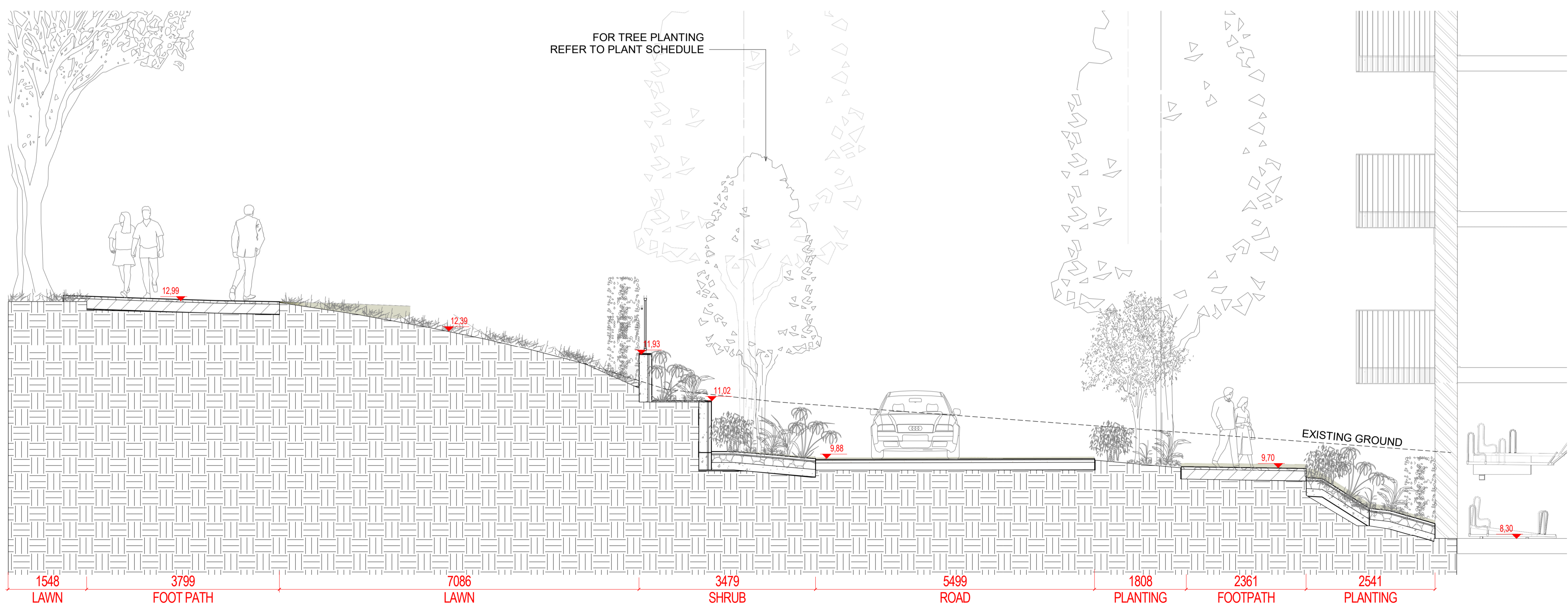
2 SECTION 45 1:50 @A1
