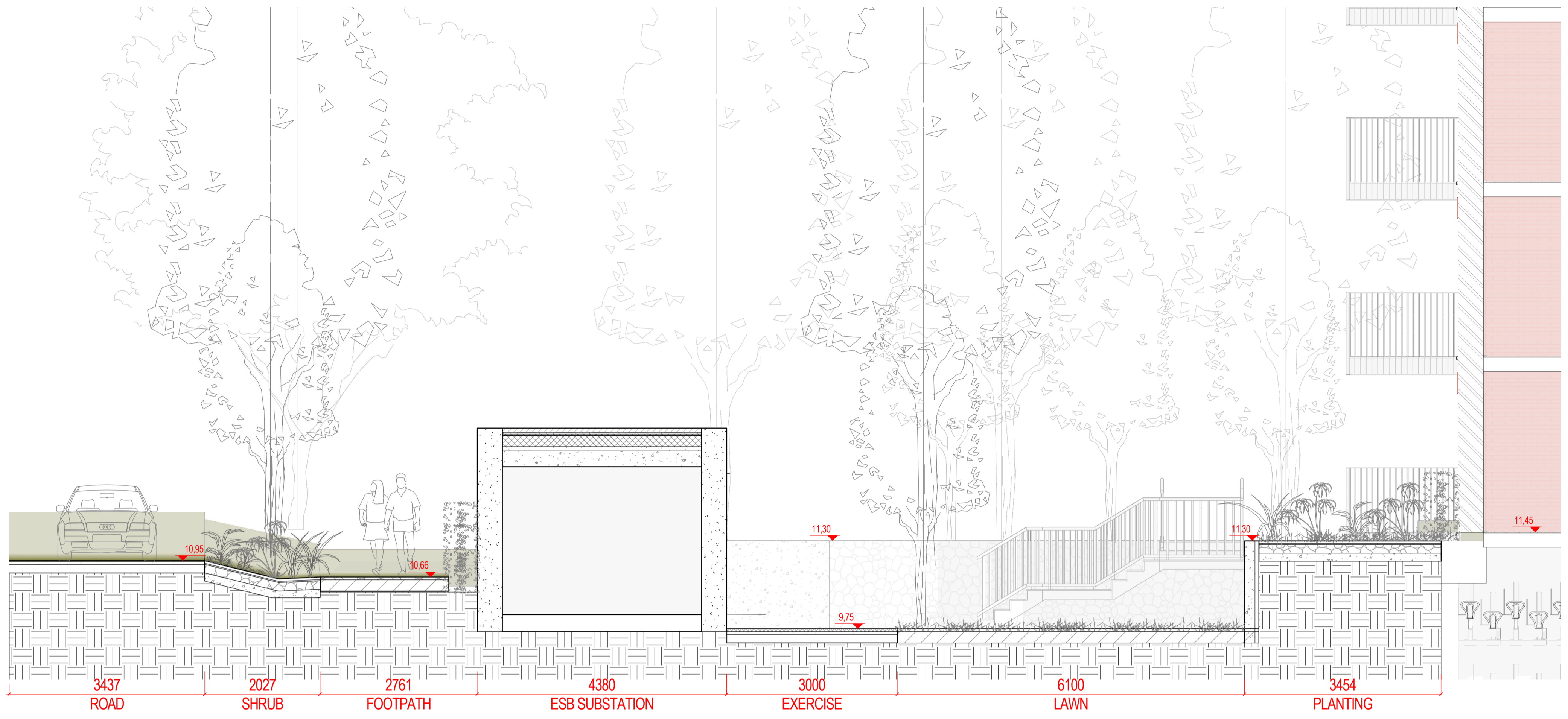
1 SECTION 44 1:50 @A1
